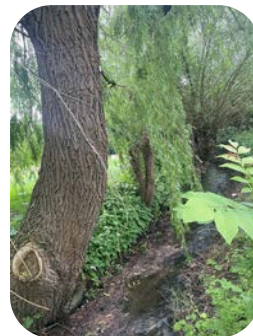
Bild 5-8: Übersichts- und Detailkarte (Quelle: www.umweltkarten-niedersachsen.de ) und Ansicht der Probestelle an der Beeke (Bickgraben).
